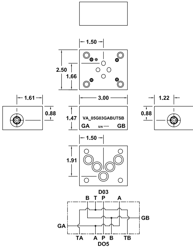
VA_05G03GAB*T**
